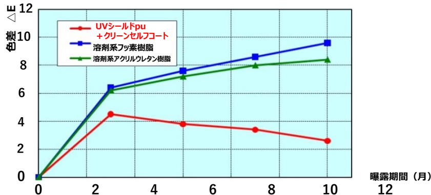
□屋外曝露汚染性 / 曝露地：大阪[堺泉北臨界工業地帯]
