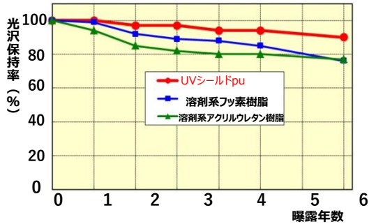
□屋外曝露による耐候性試験 / 曝露地：沖縄
