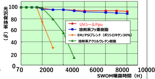
□サンシャインウェザーメーター (SWOM)による促進耐候性試験 サイクル条件：温度 (BP) 63℃、照射1時間42分+ (照射+降雨) 18分
